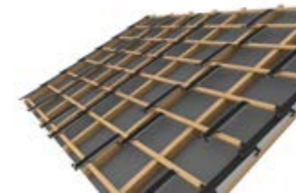
2 Fissare i ganci per il montaggio dei moduli
